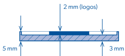
Corte A.B
